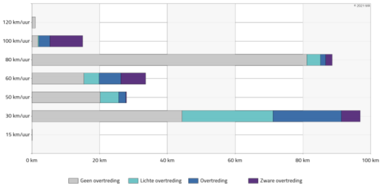
Figuur 8: Snelheidsoverschrijdingen Voerendaal per kilometer weglengte per snelheidslimiet (juli 2020)
