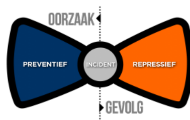
Figuur 13: Vlinderdasmodel
